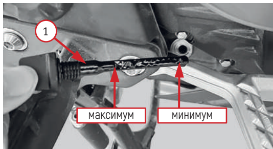
Фото 5.4. Пробка с щупом контроля уровня масла 1
