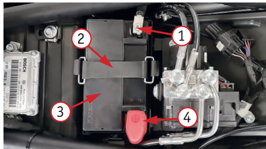
Фото 4. Аккумуляторный отсек: 1 – клемма «минус»; 2 – ремень крепления аккумуляторной батареи (АКБ); 3 – аккумуляторная батарея; 4 – колпачок клеммы «плюс»
