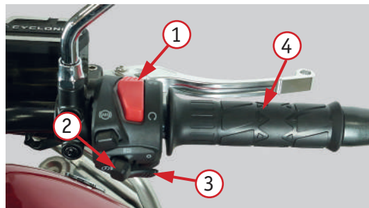
Фото 2.5. Правый комбинированный переключатель: 1 – переключатель включения/отключения питания; 2 – кнопка включения/выключения света; 3 – кнопка электростартера; 4 – ручка газа (акселератора)
