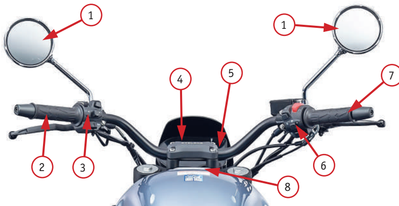
Фото 2.1. Вид руля и органов управления мотоцикла: 1- зеркало заднего вида; 2 - левая рулевая рукоятка; 3 - левый комбинированный переключатель; 4 – приборная панель; 5 - замок зажигания (под панелью); 6 - правый комбинированный переключатель; 7 - рукоятка газа (акселератор); 8 - замок крышки топливного бака
