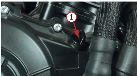
Фото 5.5. Пробка горловины для залива масла 1
