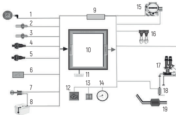
Схема 1. Схема системы EFI: 1 - датчик положения коленчатого вала; 2 - датчик кислорода L; 3 - датчик кислорода R; 4 - термодатчик двигателя; 5 - датчик температуры/давления всасываемого воздуха; 6 - выключатель нейтральной передачи; 7 - индикатор нейтральной передачи; 8 - аккумуляторная батарея; 9 - сигнализатор нештатного воздействия; 10 - модуль контроля; 11 - разъем для диагностики неисправностей/последовательный интерфейс связи; 12 - индикатор неисправности; 13 - контрольная лампа повышенной температуры двигателя; 14 - сигнал скорости вращения двигателя; 15 - датчик положения дроссельной заслонки; 16 - катушка зажигания; 17 - WCPDR регулятор давления масла; 18 - масляный насос; 19 - каталитический нейтрализатор
