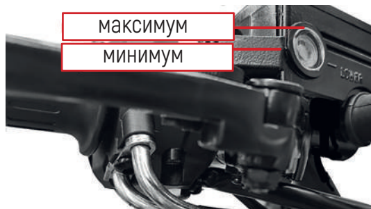
Фото 5.8. Уровень тормозной жидкости передних тормозов
