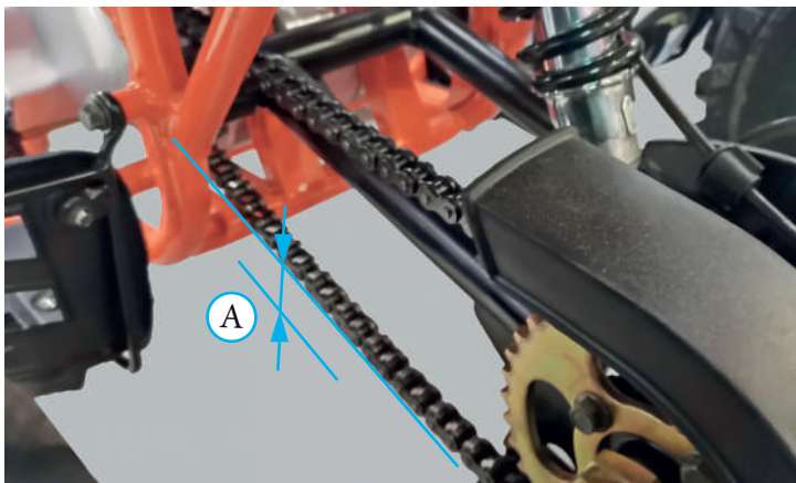
Фото 5.13. Замер провисания цепи
