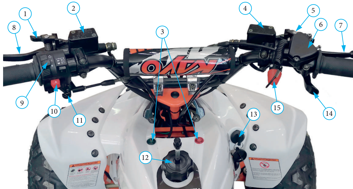
Фото 2.2. Приборы и органы управления комплекта запчастей: 1 - фиксатор стояночного заднего тормоза; 2 - бачок заднего тормоза; 3 - индикаторы (либо приборная панель); 4 - бачок переднего тормоза; 5 - фиксатор стояночного переднего тормоза; 6 - узел акселератора; 7 - рычаг переднего тормоза; 8 - рычаг заднего тормоза (либо рычаг сцепления для некоторых моделей); 9 - клавиша включения/выключения света; 10 - кнопка электростартера (вкл./выкл. двигателя); 11 - рычаг обогащения смеси (для модели TOR на карбюраторе); 12 - крышка топливного бака с сапуном; 13 - замок зажигания; 14 - рычаг акселератора; 15 - чека аварийного выключения двигателя (для MINI BULL)
