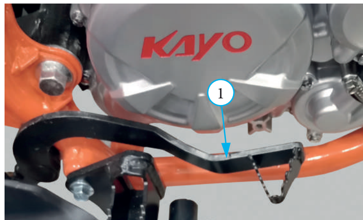
Фото 3.7. Педаль тормоза – 1
