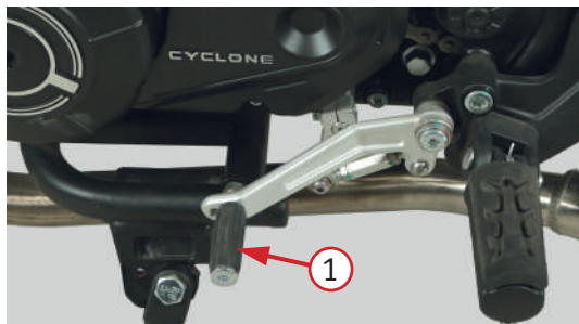
Фото 2.12. Рычаг переключения передач – 1
