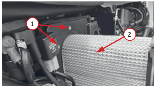
Фото 5.1. Снятие воздушного фильтра: 1 – винты крепления фильтра; 2 – фильтрующий элемент
