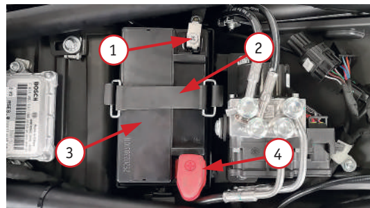
Фото 4. Аккумуляторный отсек: 1 – клемма «минус»; 2 – ремень крепления аккумуляторной батареи; 3 – аккумуляторная батарея (АКБ); 4 – колпачок клеммы «плюс»
