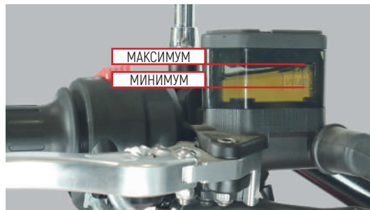
Фото 5.7. Уровень тормозной жидкости переднего тормоза
