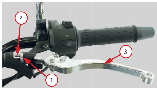
Фото 2.11. Регулировка сцепления: 1 – стопорная гайка; 2 – регулировочный винт; 3 – рычаг сцепления
