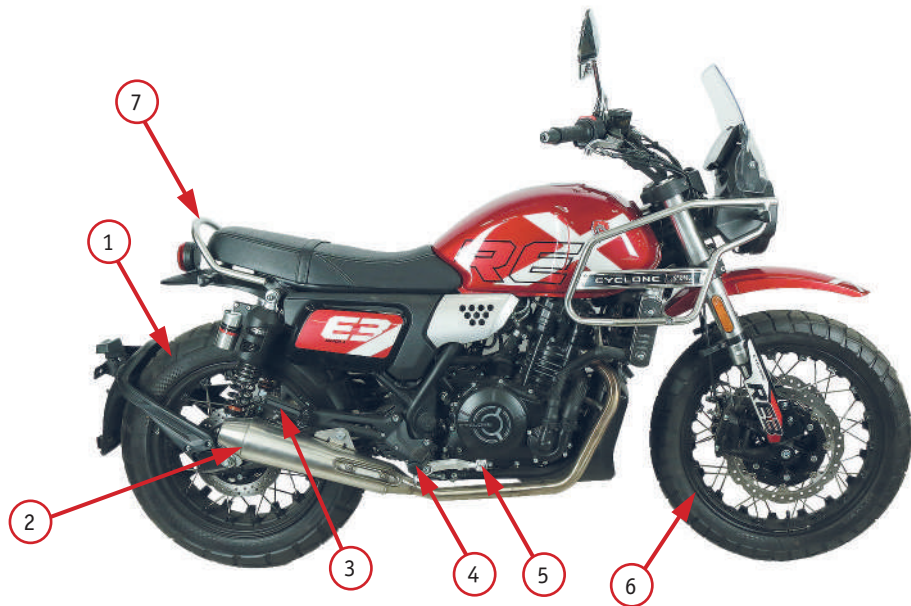
Фото 2.2. Вид справа: 1 – заднее колесо; 2 – глушитель; 3 – правая подножка пассажира; 4 – правая подножка водителя; 5 – педаль заднего тормоза; 6 – переднее колесо; 7 – поручень пассажира
