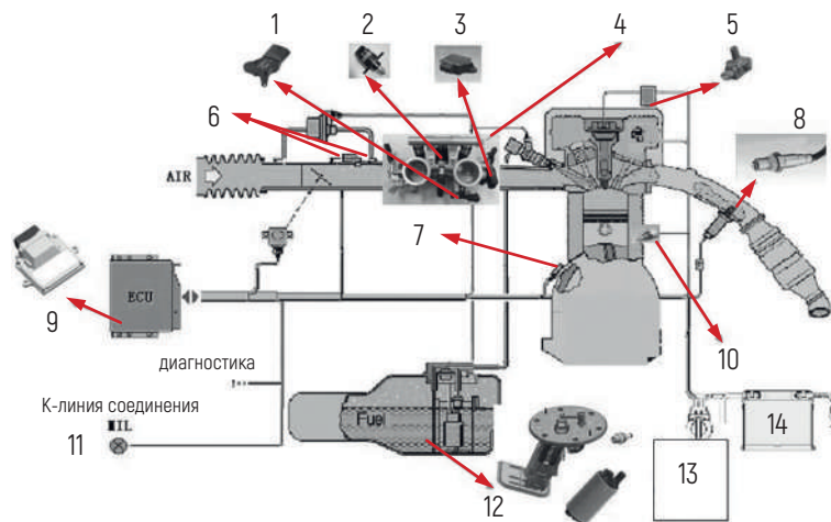
35 Схема 1. Схема системы EFI: 1 – датчик давления / температуры поступающего воздуха; 2 – регулятор холостого хода; 3 – датчик положения дроссельной заслонки; 4 – топливная рейка в сборе; 5 – катушка зажигания; 6 – корпус дроссельной заслонки; 7 – датчик положения коленчатого вала; 8 – датчик кислорода; 9 – электронный блок управления двигателем (ЭБУ); 10 – датчик температуры двигателя; 11 – лампа сигнализации о неисправности; 12 – топливный насос с кронштейном; 13 – насос топливный / клапан регулировки давления / фильтр тонкой очистки; 14 – аккумуляторная батарея (АКБ)
