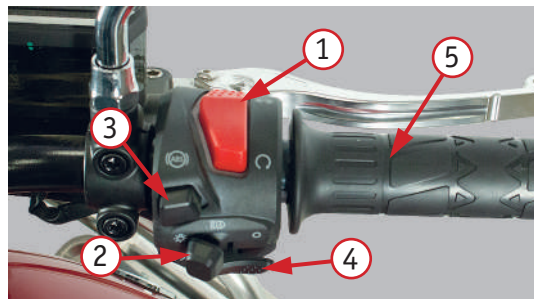
Фото 2.5. Правый комбинированный переключатель: 1 – переключатель включения/отключения питания; 2 – кнопка включения/выключения света; 3 – кнопка отключения ABS; 4 – кнопка электростартера; 5 – ручка газа (акселератора)
