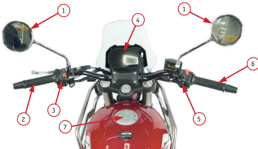
Фото 2.1. Вид руля и органов управления мотоцикла: 1 – зеркало заднего вида; 2 – левая рулевая рукоятка; 3 – левый комбинированный переключатель; 4 – приборная панель; 5 – правый комбинированный переключатель; 6 – рукоятка газа (акселератор); 7 – замок крышки топливного бака
