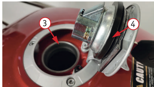
Фото 2.6. Топливный бак: 1 – защитная створка замочной скважины топливного бака; 2 – замочная скважина топливного бака; 3 – горловина топливного бака; 4 – крышка топливного бака в открытом виде
