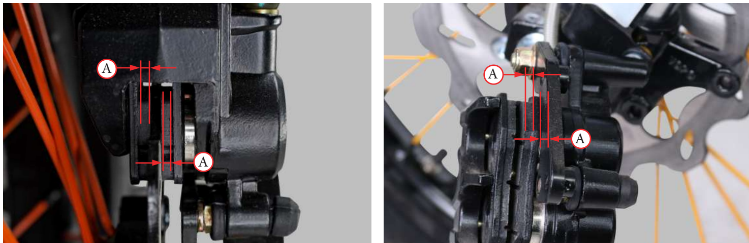
Фото 5.19. Толщина тормозных колодок - А.
