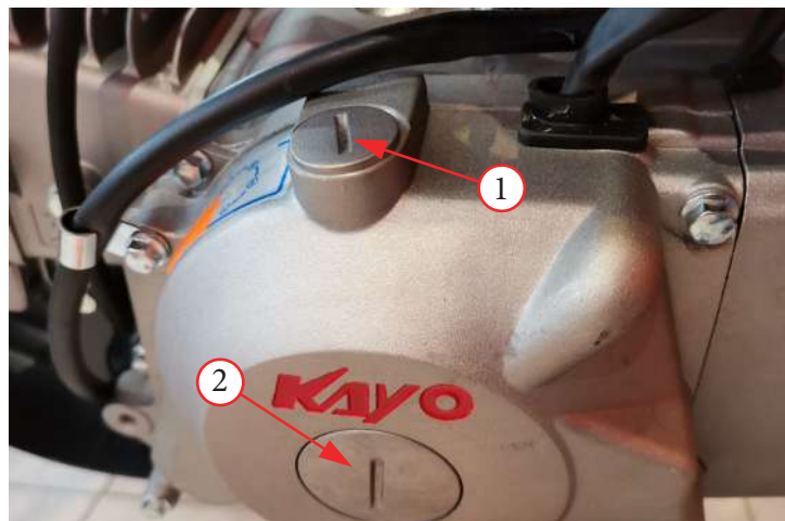
Фото 5.33. Пробки: 1 – окна с метками на маховике; 2 – к креплению маховика коленчатого вала.
