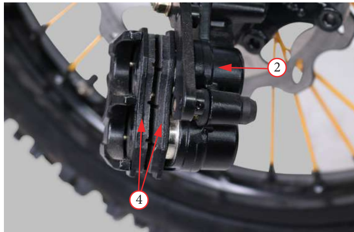
Фото 5.21. Замена передних тормозных колодок.
