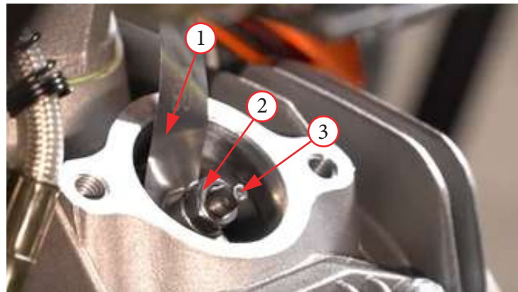
Фото 5.37. Регулировки теплового зазора: 1 – шуп; 2 – контргайка; 3 – регулировочный винт.
