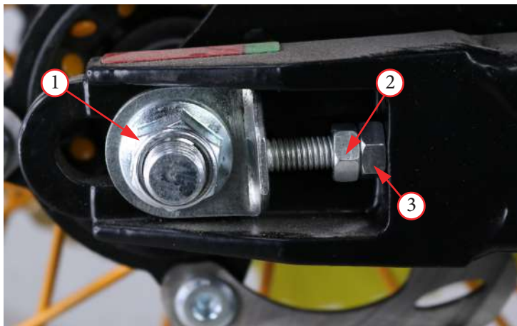
Фото 5.28. Замена цепи.
