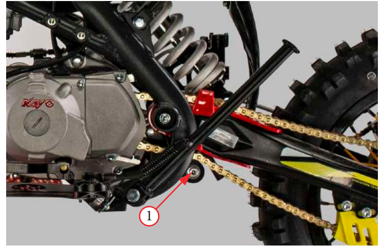
Фото 5.25. Ролик натяжения цепи – 1, слайдер-успокоитель – 2.
