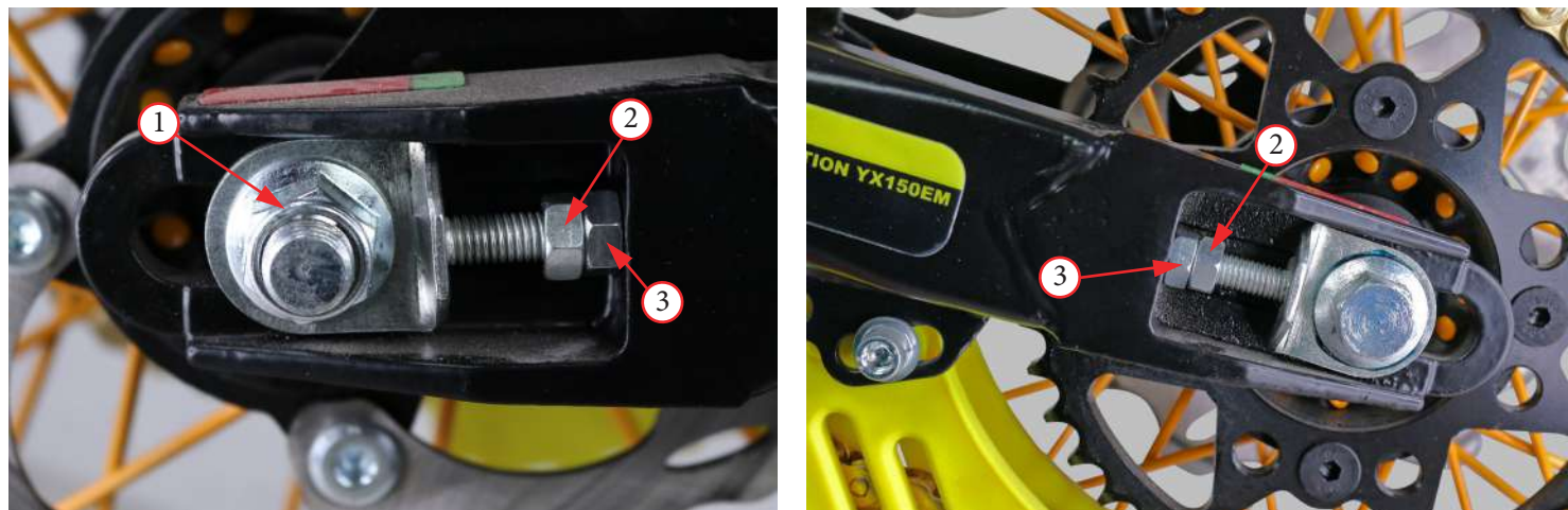
Фото 5.26. Регулировка натяжения цепи.
